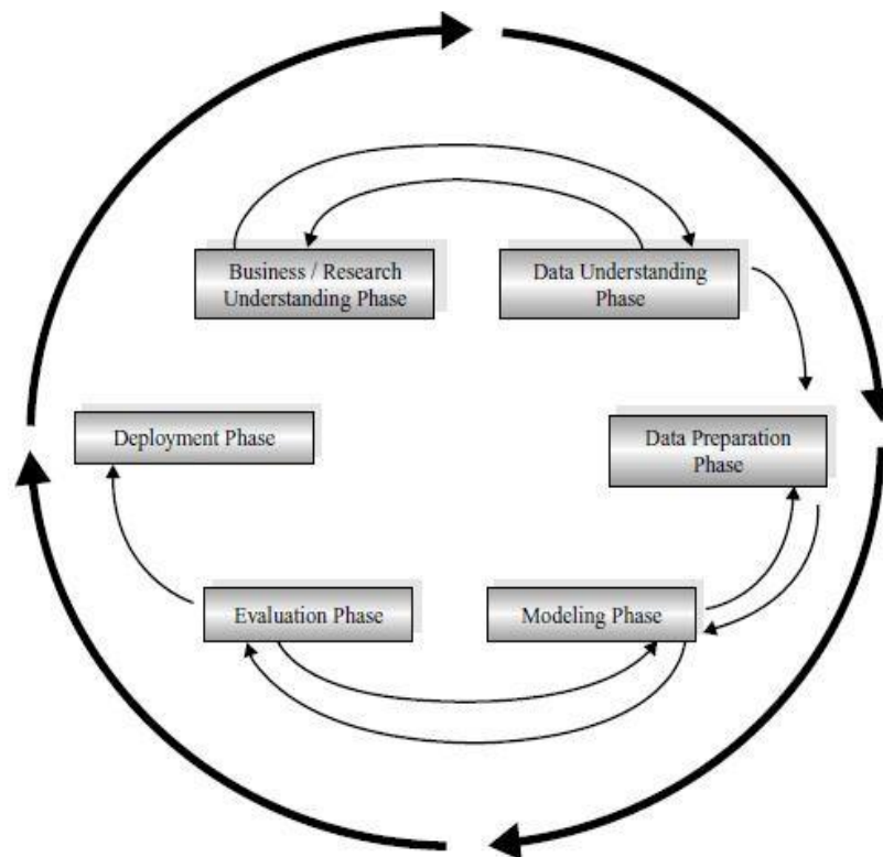
Gambar 2 Tahapan Metodologi CRISP-DM oleh Larose (Setiawan, 2016)
